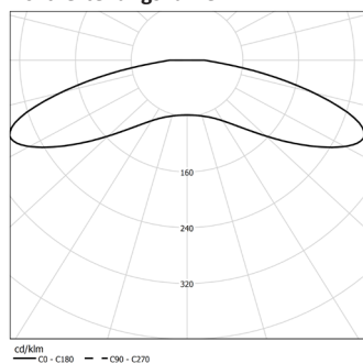
Lichtverteilungskurve
