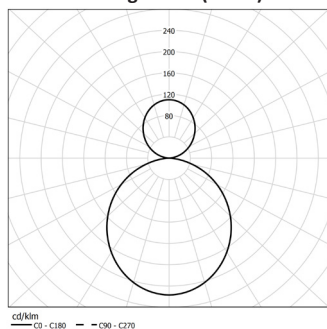
Lichtverteilungskurve (B & D)
