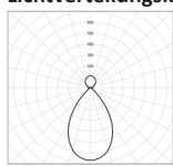
Lichtverteilungskurve (B & D)
